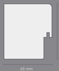
Randholz Bordure de bois
